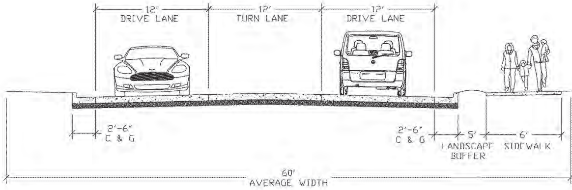
TYPICAL ROAD SECTIONS SCALE: N.T.S.
